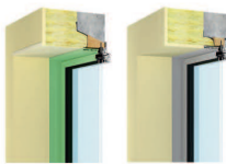
Isolation thermique par l'extérieur (ITE)
